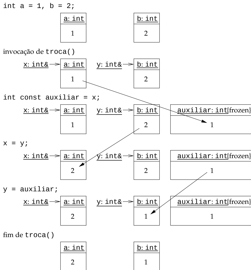
Figura 3.2: Diagramas com evolução do estado do programa que invoca o procedimento troca() entre cada instrução.
