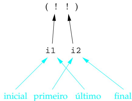
Figura 10.2: Definição de iteradores e itens canônicos de uma lista vazia. Note-se que os iteradores primeiro e último trocam as suas posições usuais. Decorre daqui que são estes iteradores que se definem à custa dos iteradores início e fim, e não o contrário, como se sugeriu atrás.
