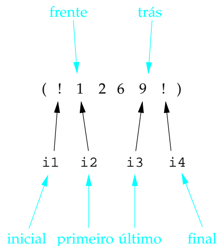
Figura 10.1: Definição de iteradores e itens canônicos das listas. Representam-se por um ponto de exclamação os itens fictícios da lista. Os iteradores primeiro ( i2 ) e último ( i3 ) referenciam respectivamente os itens na frente e na traseira da lista. Os iteradores início ( i1 ) e fim ( i4 ) são definidos como sendo respectivamente anterior ao primeiro e posterior ao último.
