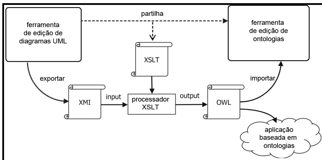
Figura 2 - Conversão usando XSLT (Gašević et al. , 2004)
