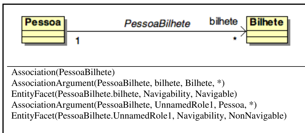
Figura 5 - Conversão de uma associação e respectivos membros
