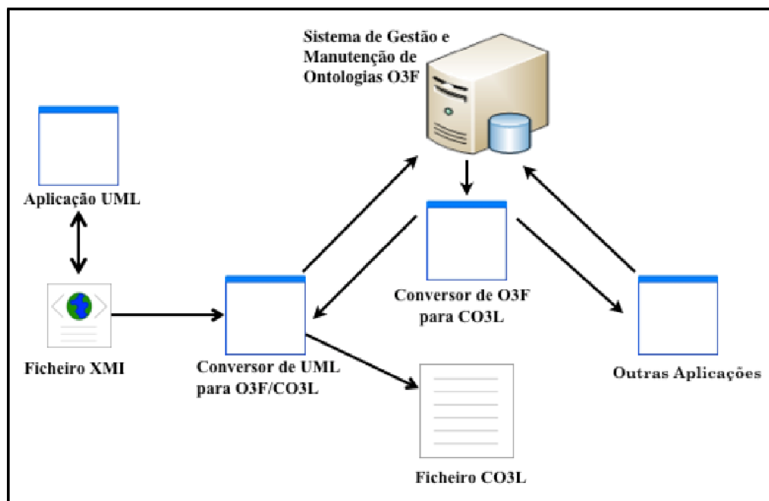
Figura 12 - Arquitectura geral do sistema
