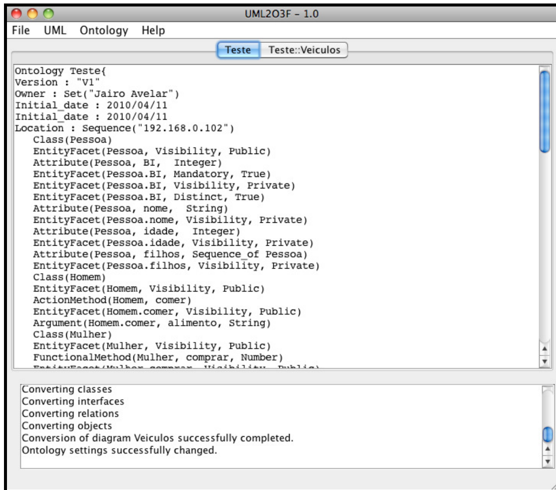
Figura 13 - Conversor de UML para O3F e CO3L
