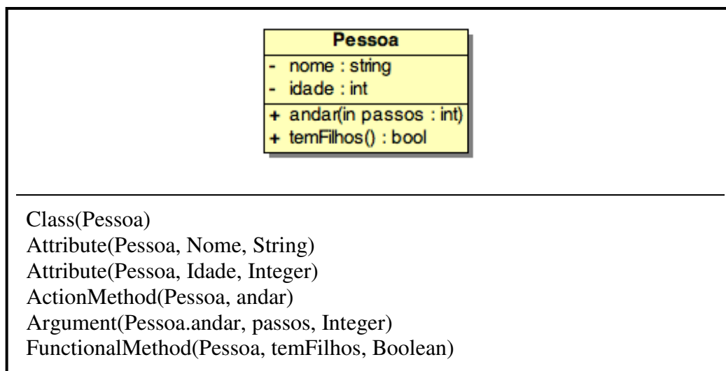
Figura 4 – Conversão de uma classe e respectivas propriedades
