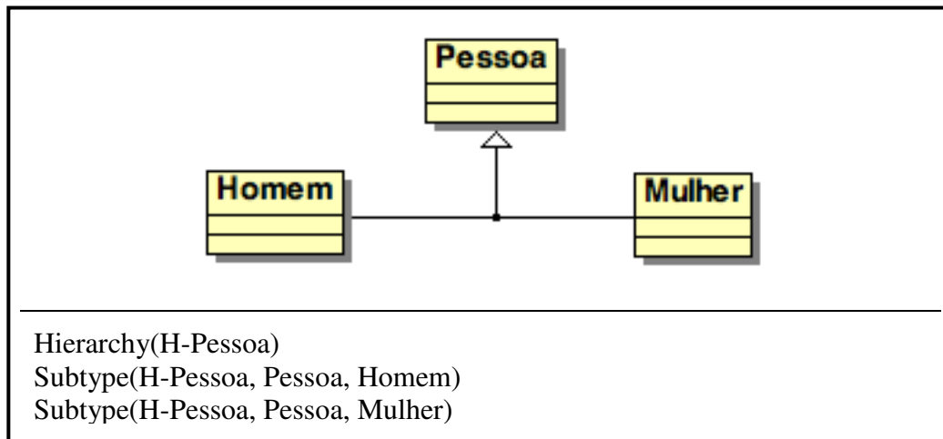
Figura 8 - Conversão de uma generalização
